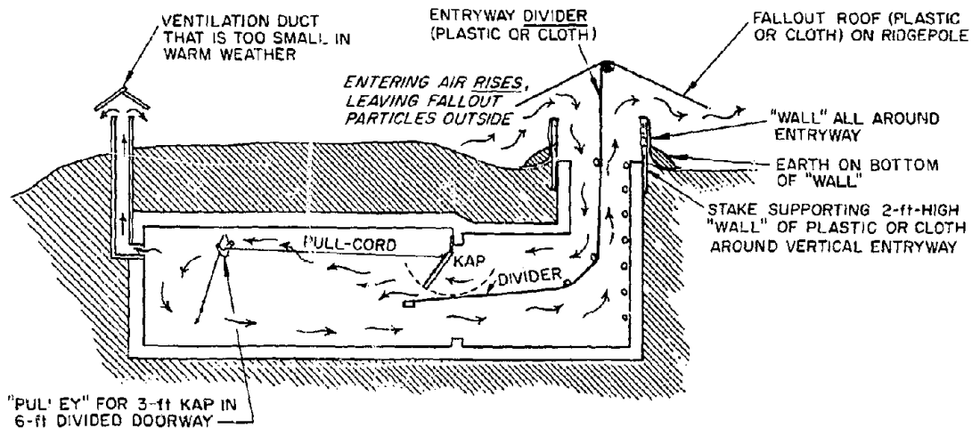
Fig. B-15. Use of air divider.
